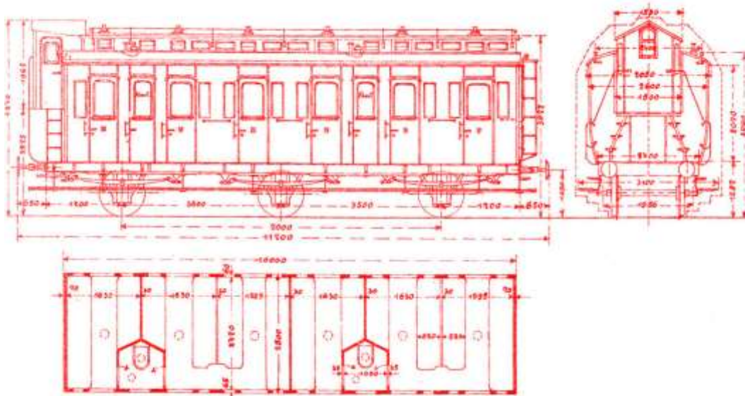
Skizze 98 C3 nach Blatt 1h 9 von 1904
