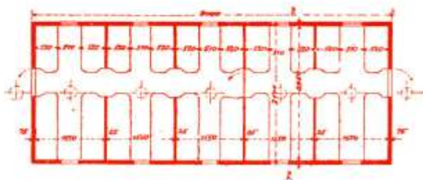
Skizze 18 Ci nach Blatt 2 der Normalien von 1883/84 (ohne Abort)
